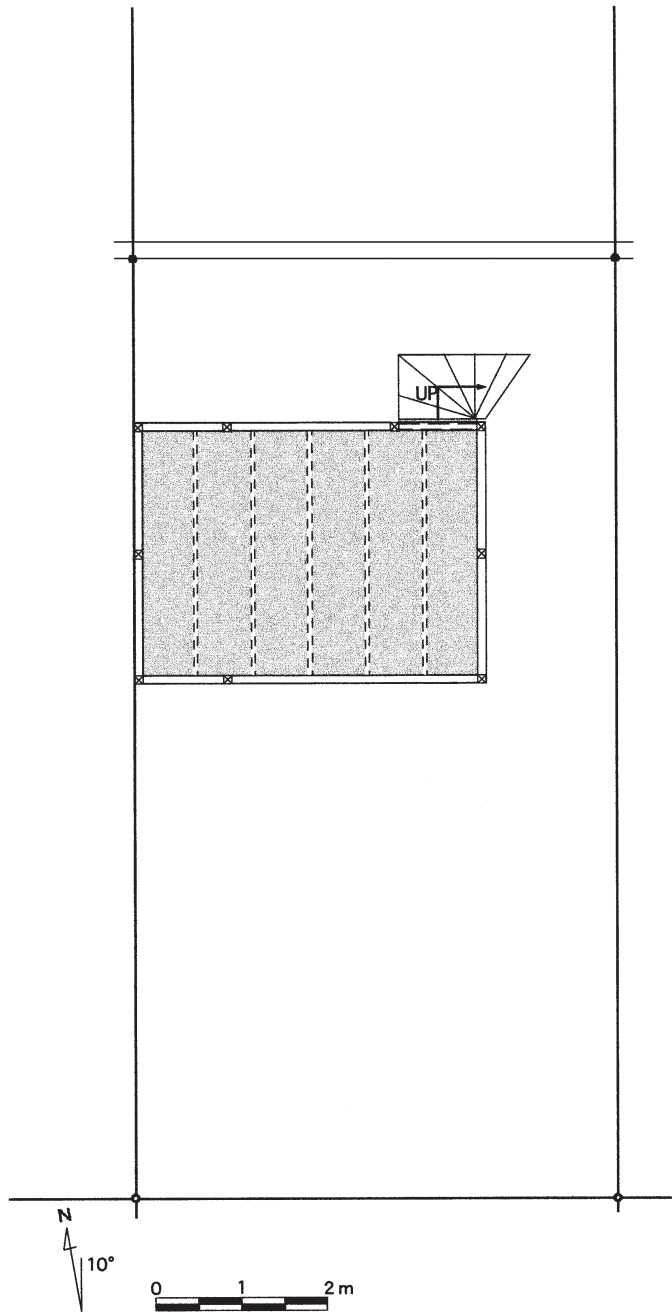
図 1-3 大村しげの住んだ町家（地階） 佐藤浩司氏の調査図をもとに作成
