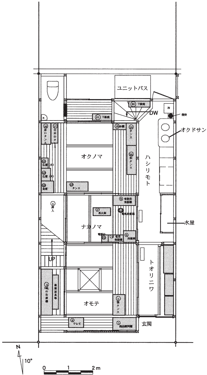
図 1-1 大村しげの住んだ町家 (1階) 佐藤浩司氏の調査図をもとに作成
